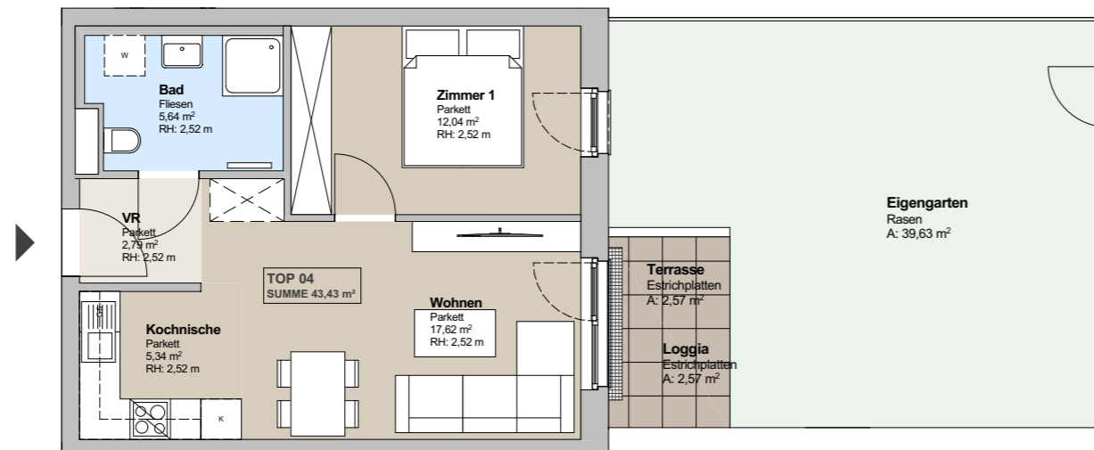
Erdgeschoß M: 1: 100
