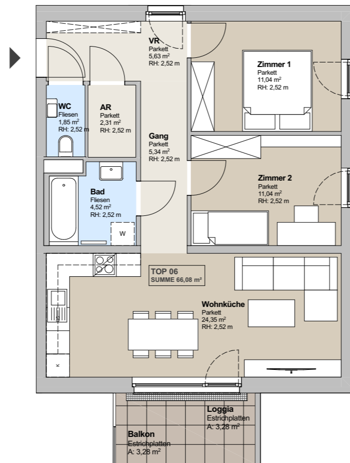
1. Obergeschoß M: 1: 100
