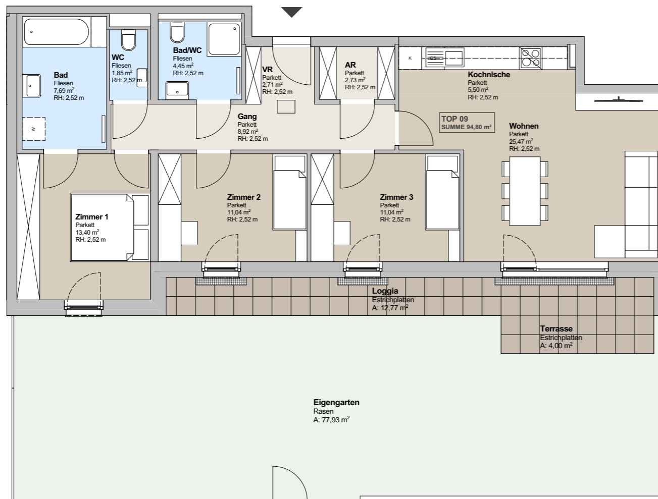
1. Obergeschoß M: 1: 100
