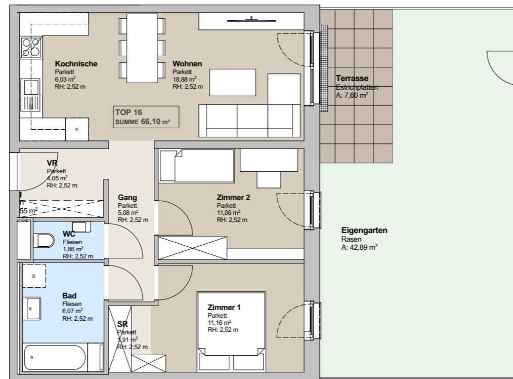
1. Obergeschoß M: 1: 100
