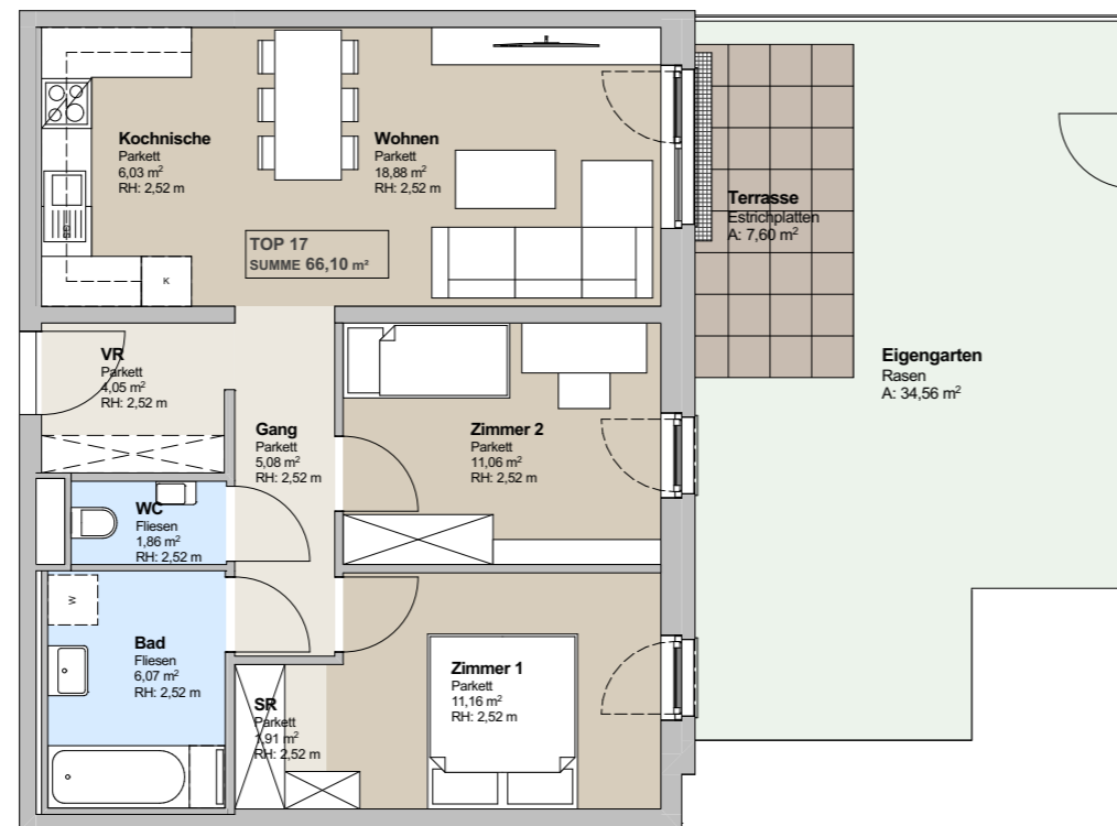
1. Obergeschoß M: 1: 100
