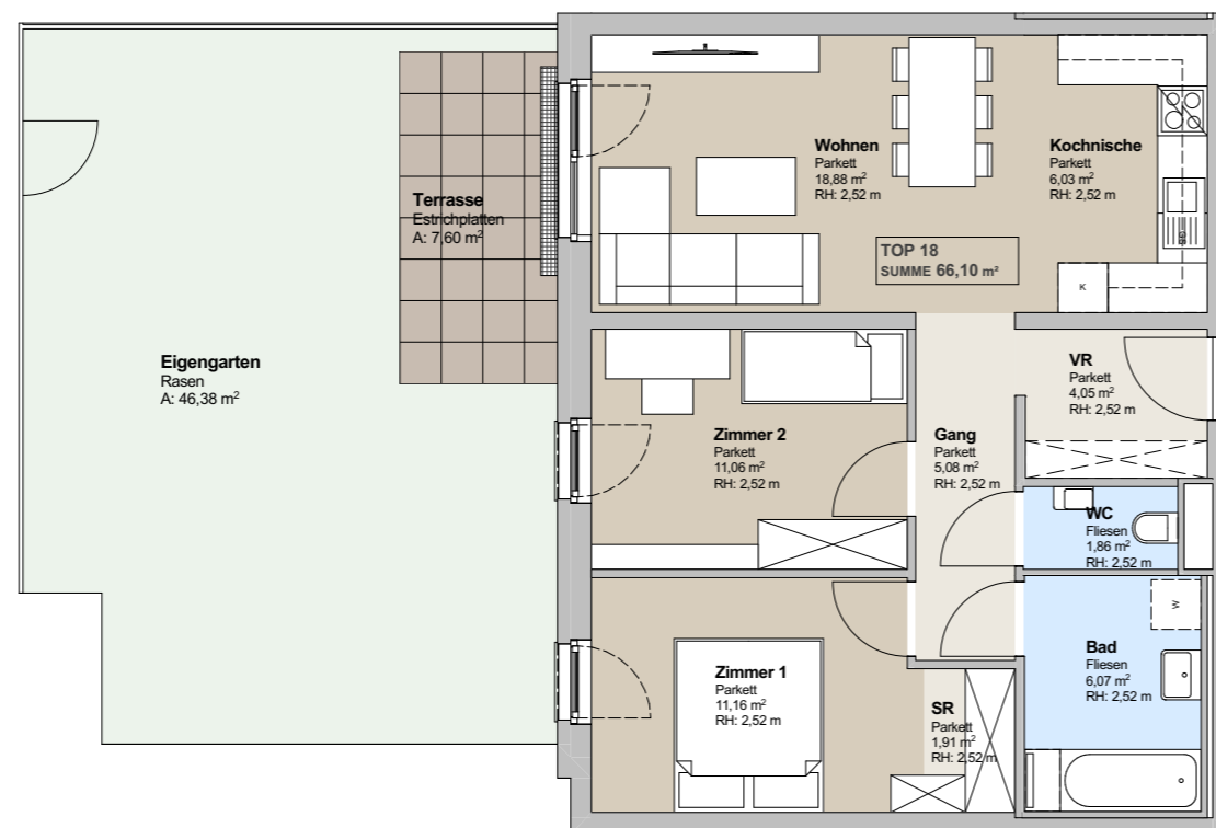
1. Obergeschoß M: 1: 100
