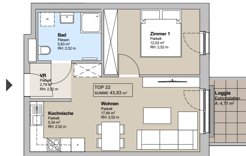
1. Obergeschoß M: 1: 100
