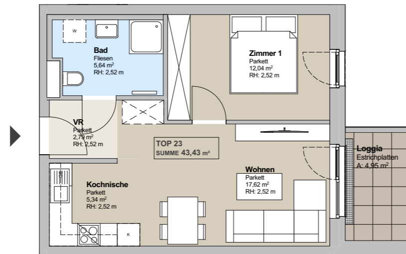
1. Obergeschoß M: 1: 100
