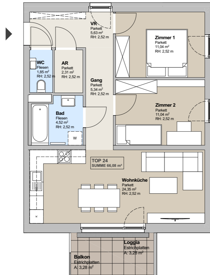
2. Obergeschoß M: 1: 100
