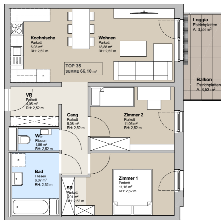
2. Obergeschoß M: 1: 100
