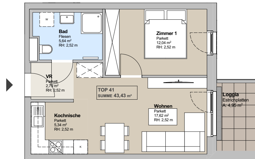
2. Obergeschoß M: 1: 100
