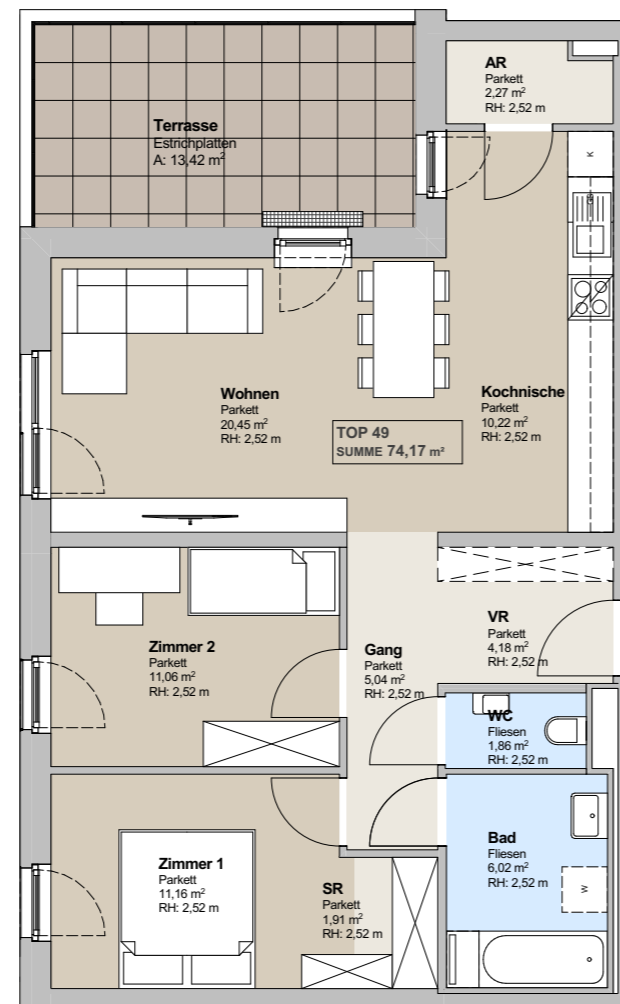
3. Obergeschoß M: 1: 100
